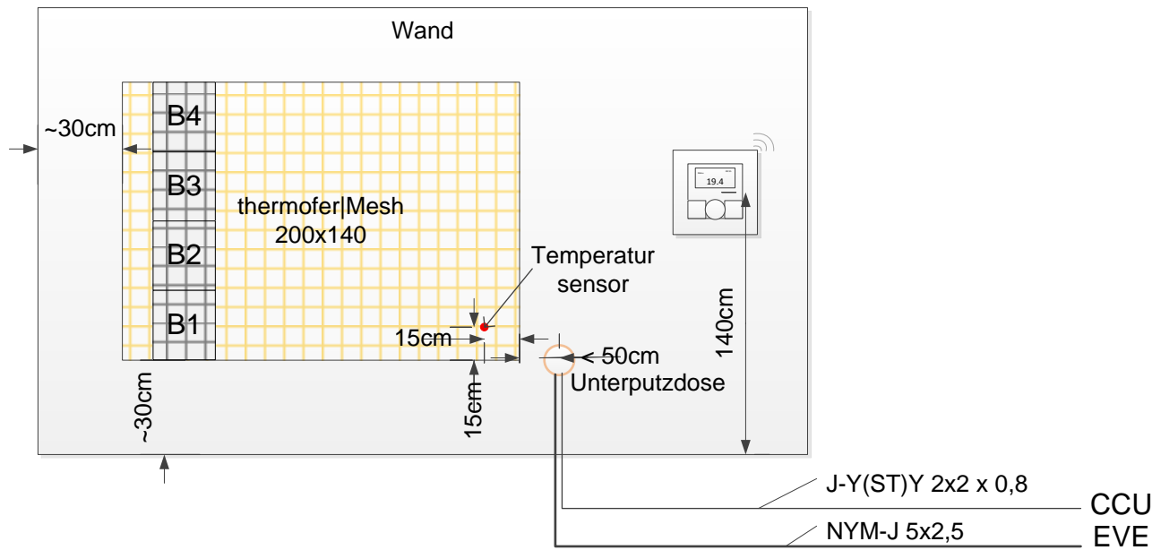
Größenvarianten thermofer|Mesh
