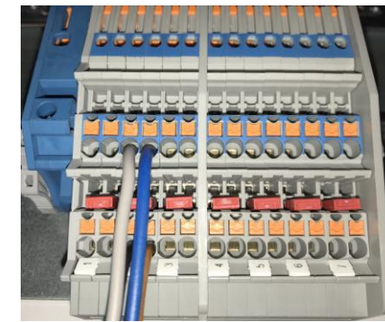
Anschlussblock in EVE
